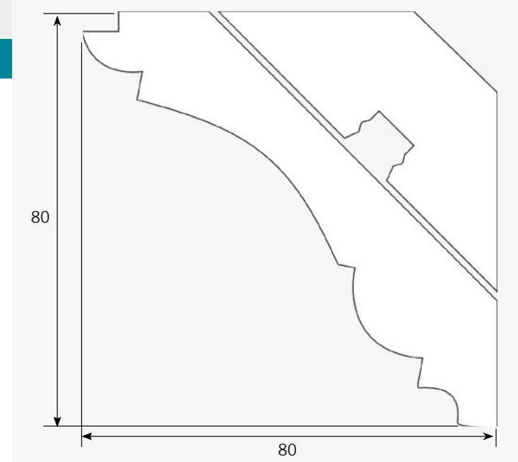
80/80 Klicksystem
