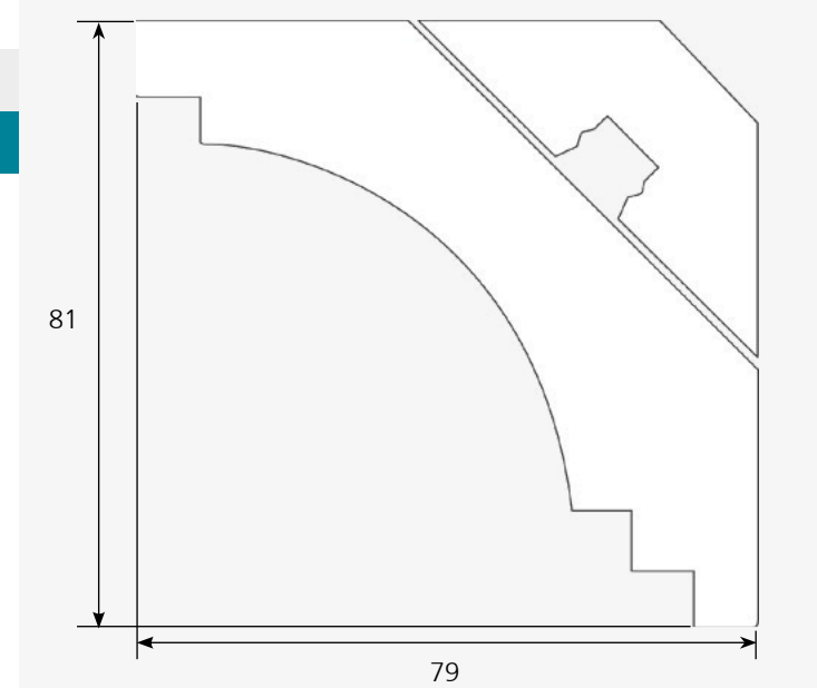
79/81 Klicksystem
