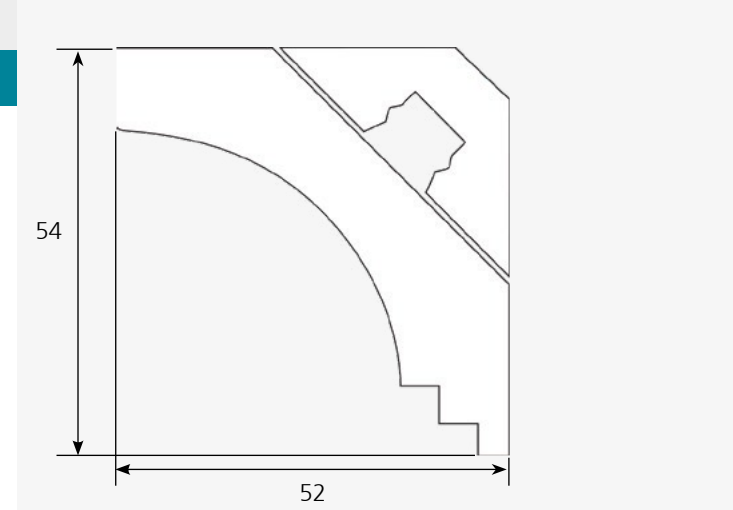
52/54 Klicksystem
